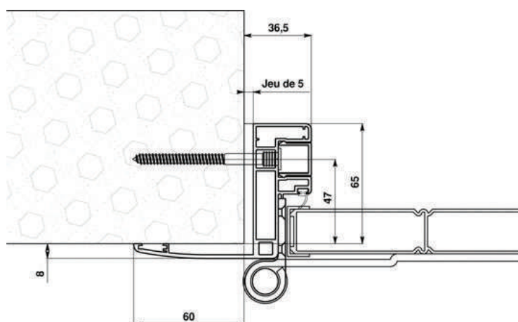
Coupe pré-cadre vue du dessus
