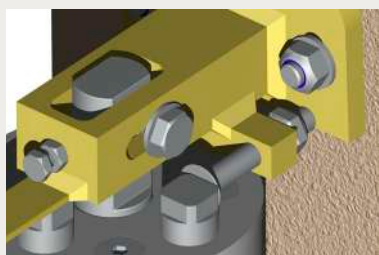
Butées internes pour ne pas déformer le portail
