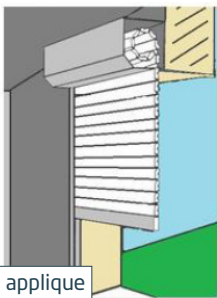
Pose en applique extérieure
