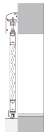
Simple voie sur terrasse
