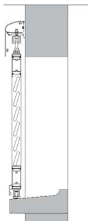
Simple voie sur appui
