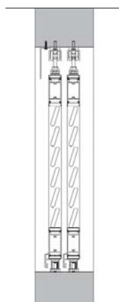
Double voie sous linteau
