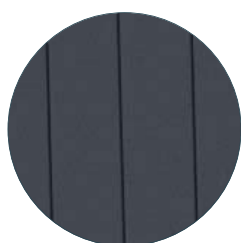
Nervure
